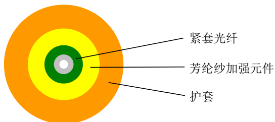
单芯圆形室内光缆
